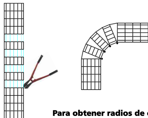
CURVA DE 90°
