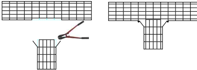
TEE
